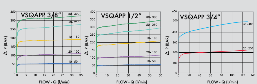
PRESSIONE/PORTATA PRESSURE/FLOW
